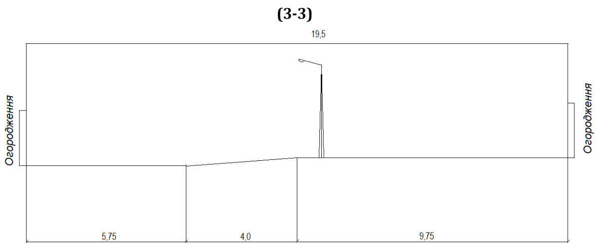
Рис.3. Існуючий поперечний профіль вул. Шумська
