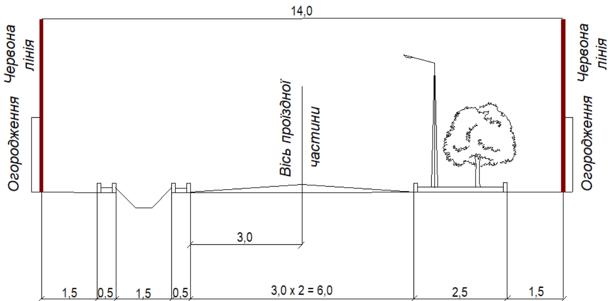
Рис.17. Прогнозовані поперечні профілі вул. Вишнева
