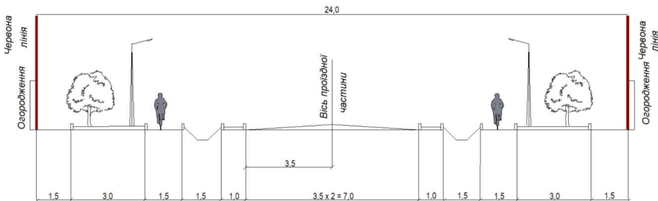
Рис.13. Прогнозовані поперечні профілі вул. Центральна
