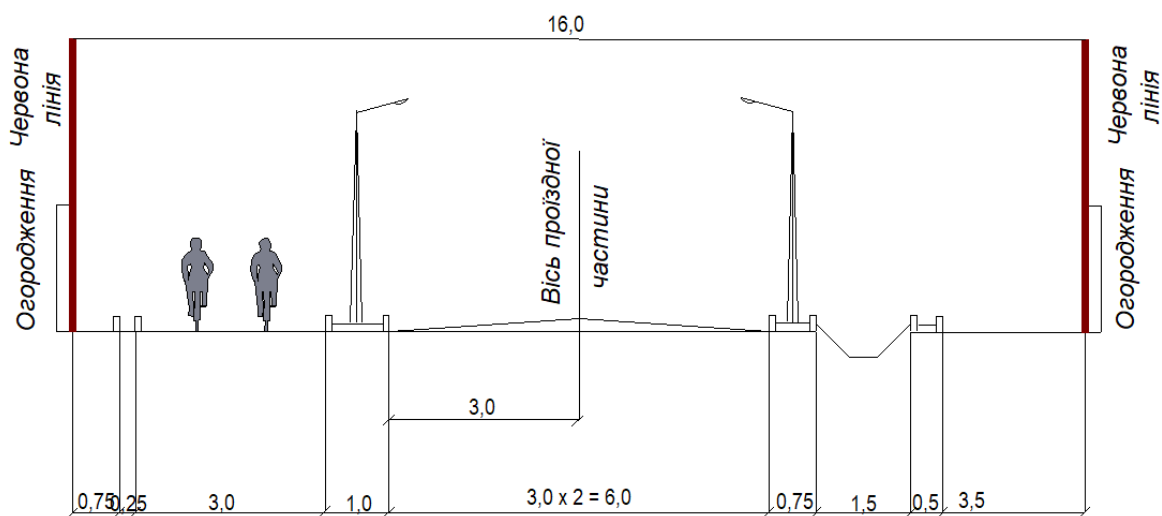
Рис.19. Прогнозовані поперечні профілі вул. Миру
