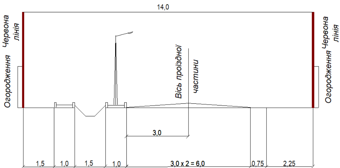
Рис.21. Прогнозовані поперечні профілі вул. Набережна
