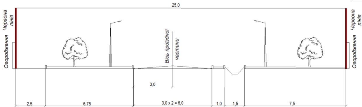
Рис.20. Прогнозовані поперечні профілі вул. Лісова
