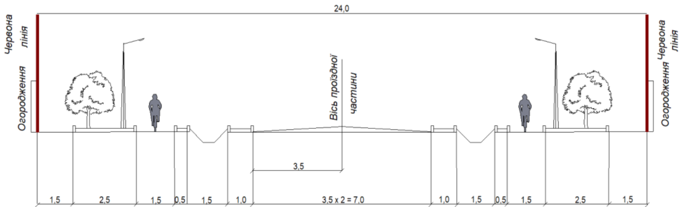
Рис.14. Прогнозовані поперечні профілі вул. Центральна
