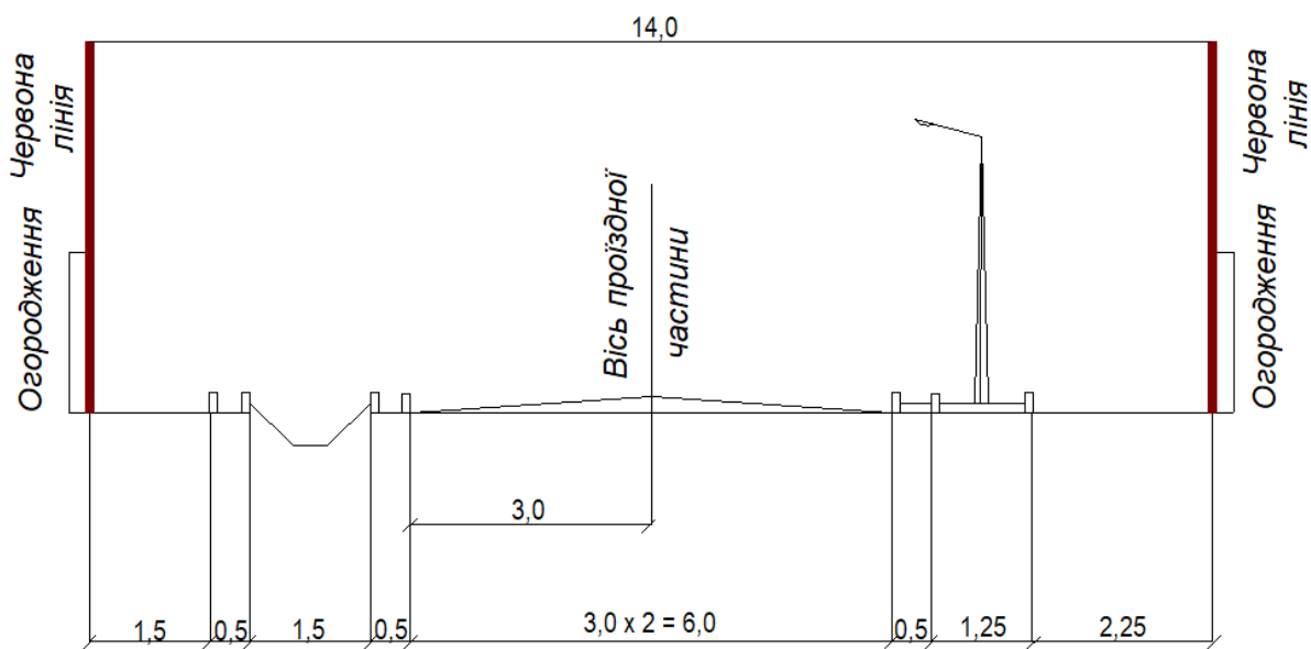
Рис.22. Прогнозовані поперечні профілі вул. 1 Лінія
