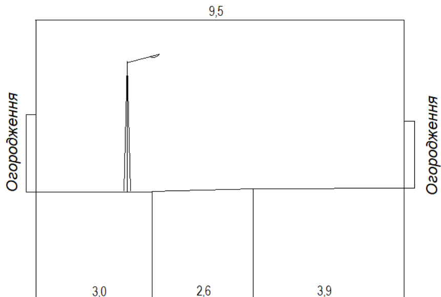
Рис.12. Існуючий поперечний профіль вул. Дружби
