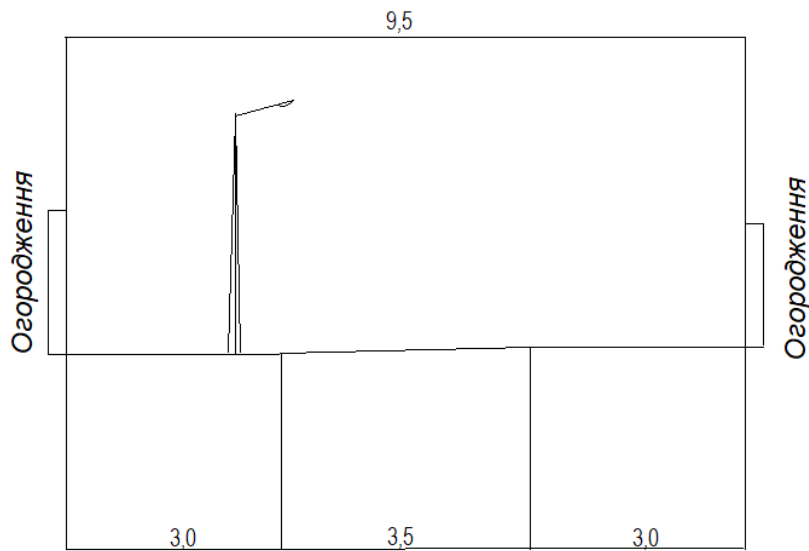
Рис.7. Існуючий поперечний профіль вул. Набережна
