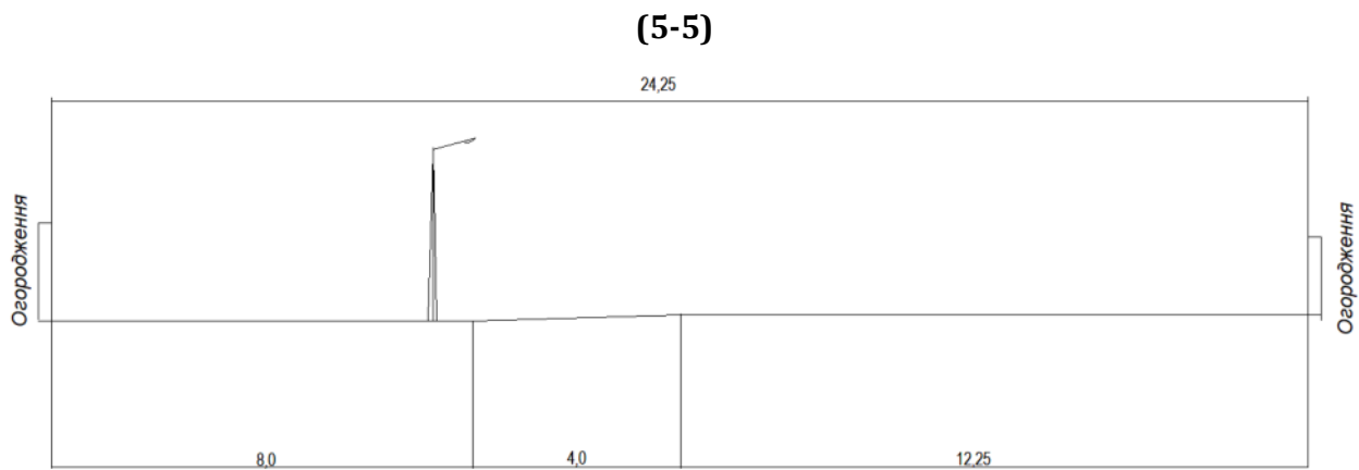
Рис.5. Існуючий поперечний профіль вул. Миру
