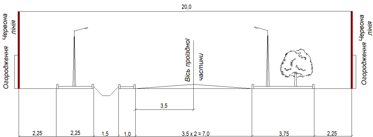
Рис.24. Прогнозовані поперечні профілі вул. 3 Лінія
