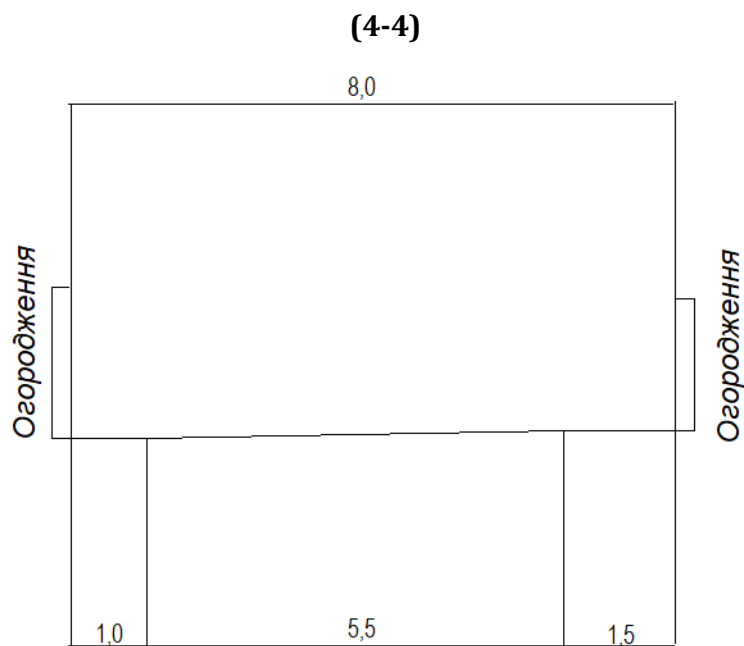
Рис.3. Існуючий поперечний профіль вул. Шумська
