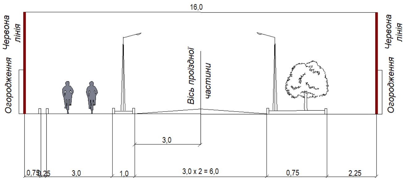
Рис.29. Прогнозовані поперечні профілі вул. Проектна 3
