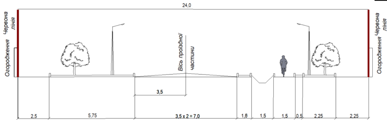
Рис.17. Прогнозовані поперечні профілі вул. Вишнева
