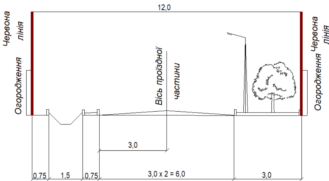
Рис.24. Прогнозовані поперечні профілі вул. 3 Лінія
