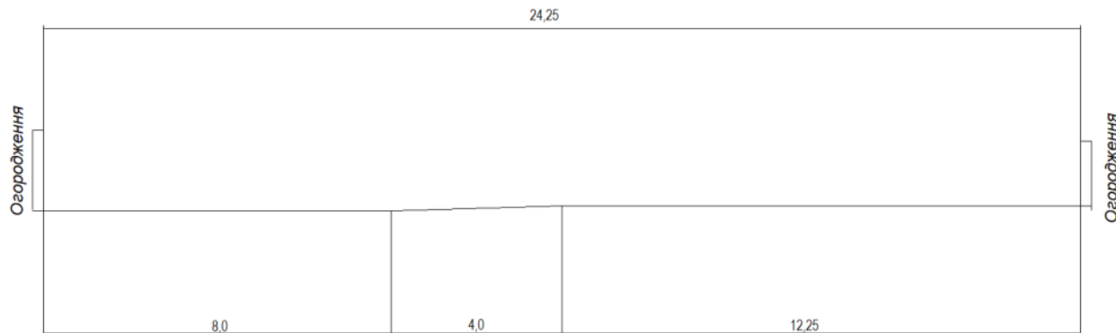
Рис.6. Існуючий поперечний профіль вул. Лісова
