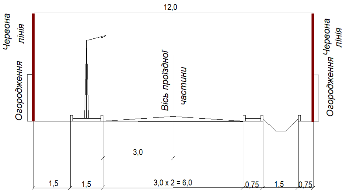
Рис.32. Прогнозовані поперечні профілі вул. Проектна 6
