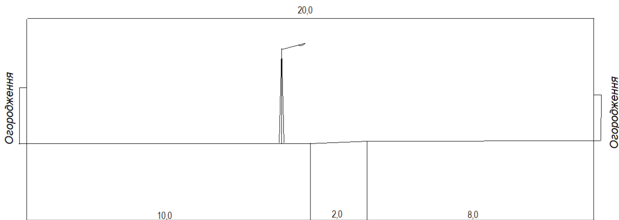
Рис.10. Існуючий поперечний профіль вул. 3 лінія
