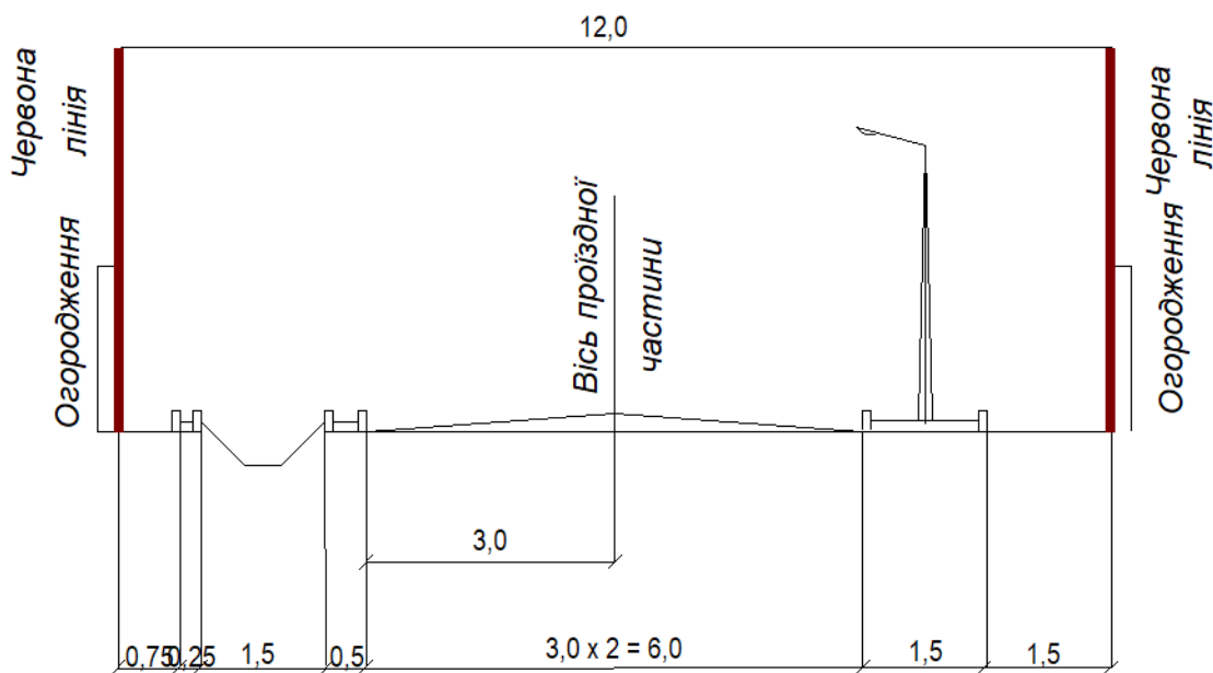
Рис.27. Прогнозовані поперечні профілі вул. Проектна 1
