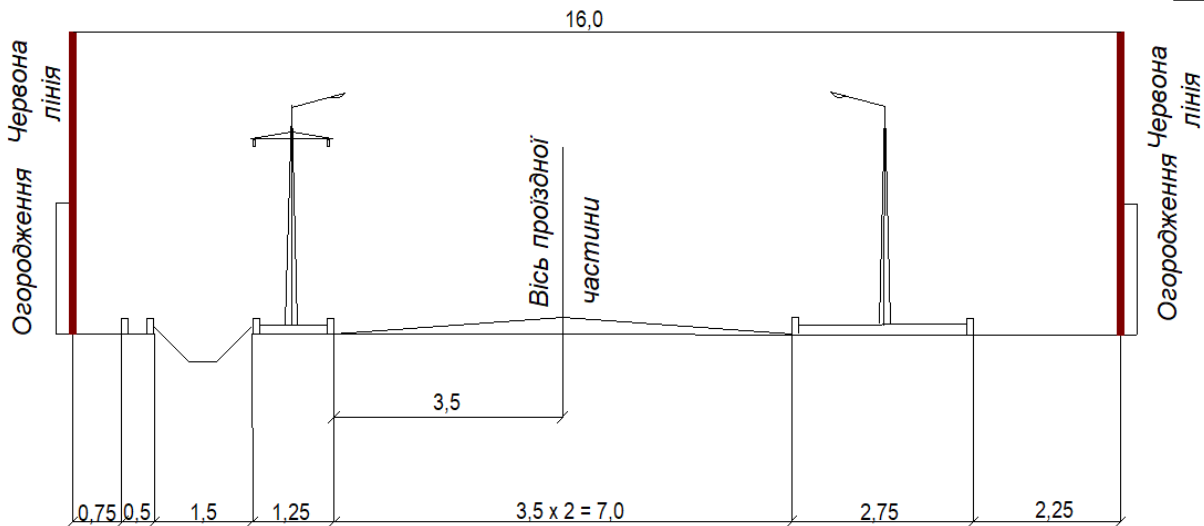
Рис.23. Прогнозовані поперечні профілі вул.2 Лінія
