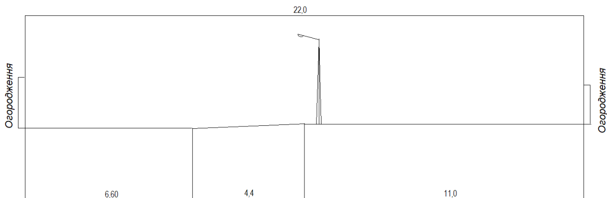
Рис.8. Існуючий поперечний профіль вул. 1 Лінія
