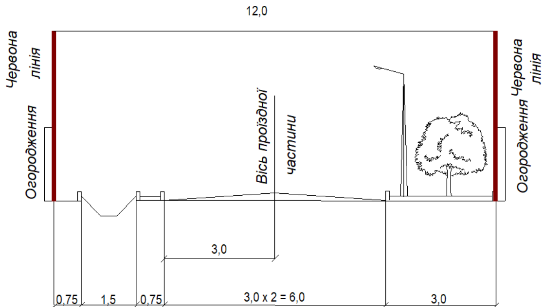
Рис.33. Прогнозовані поперечні профілі вул. Проектна 7
