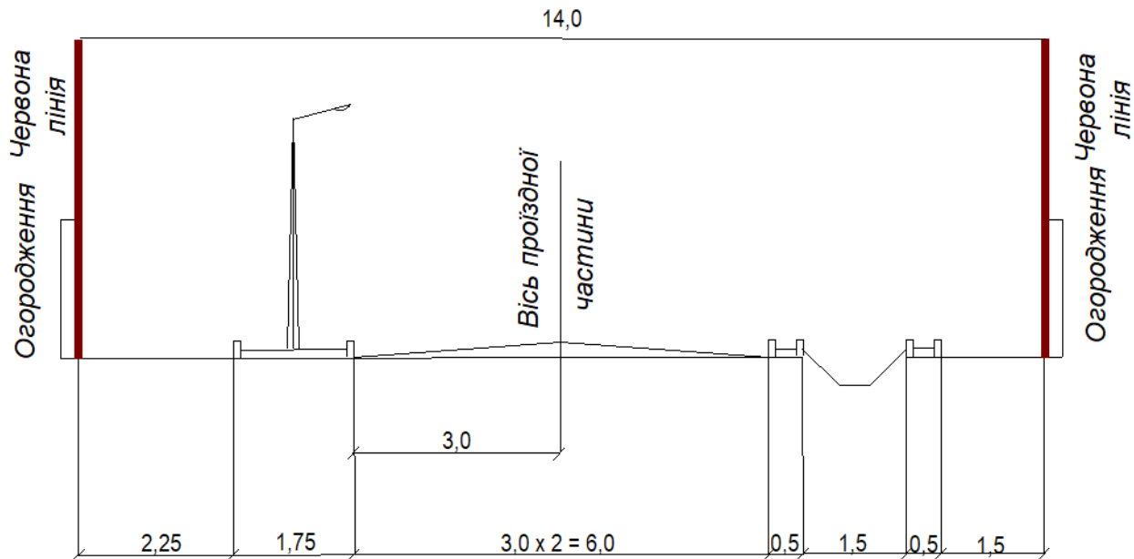
Рис.26. Прогнозовані поперечні профілі вул. Дружби
