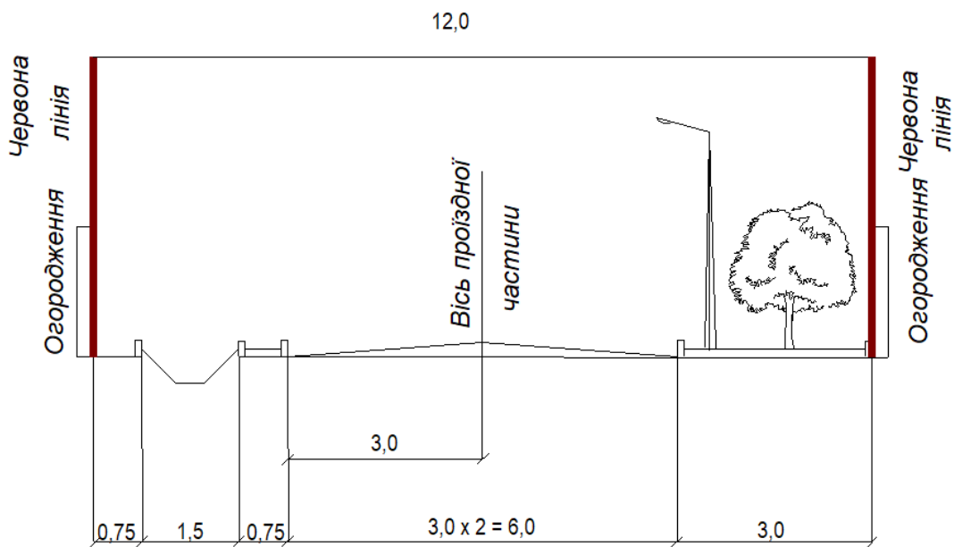
Рис.30. Прогнозовані поперечні профілі вул. Проектна 4
