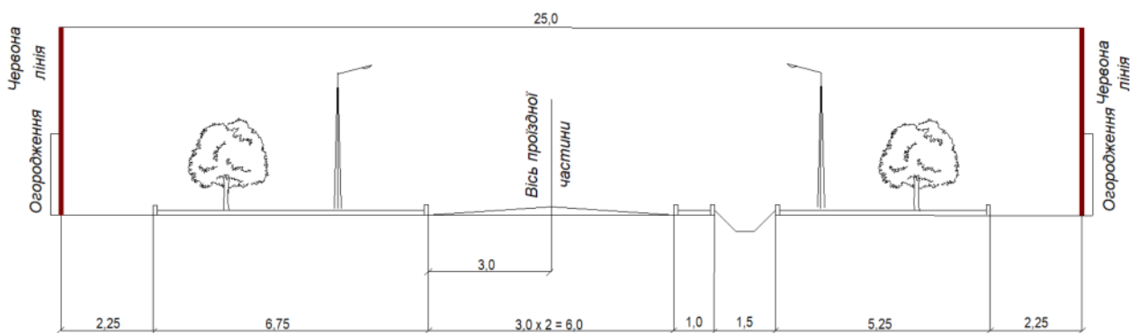
Рис.34. Прогнозовані поперечні профілі вул. Проектна 8
