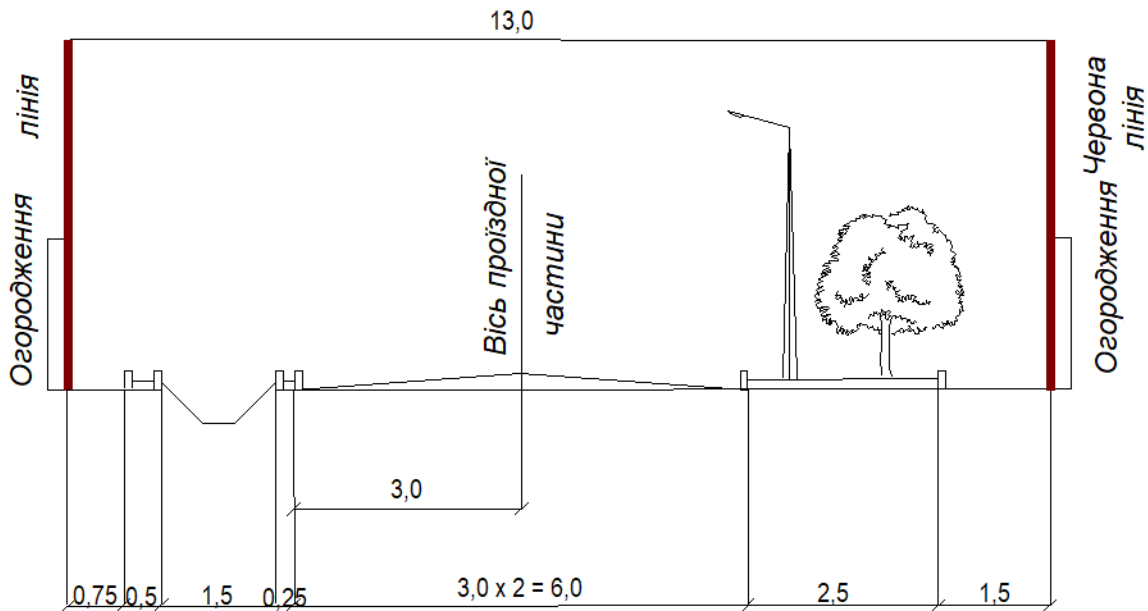
Рис.31. Прогнозовані поперечні профілі вул. Проектна 5
