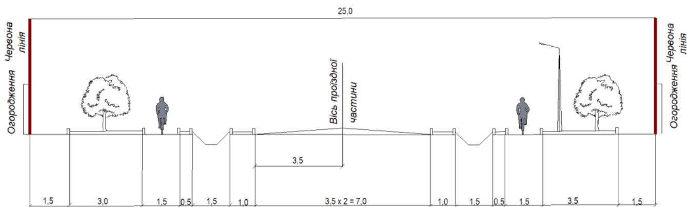
Рис.28. Прогнозовані поперечні профілі вул. Проектна 2
